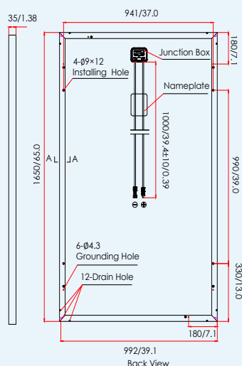
DIMENSIONS OF PV MODULE unit:mm/inches
